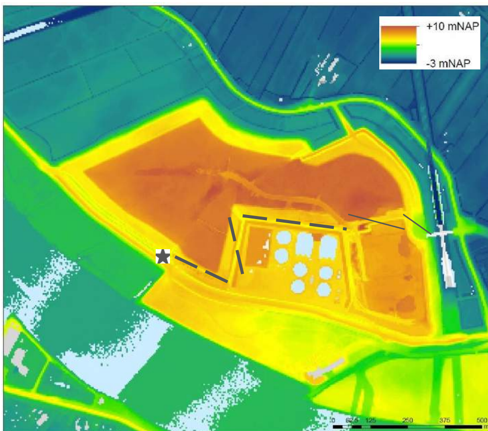
Figuur 4: Hoogtekarta. De watergang is indicatief aangegeven met de grijze stippellijn, de locatie van het gemaal met de ster en de toegangsroute die gebruikt wordt voor het onderhoud aan de watergang met de dunne grijze lijn. (Bron: AHN2, Nationaal Georegister)
